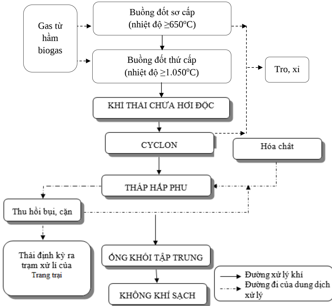
Hình 3.3. Sơ đồ công nghệ hệ thống xử lý khí thải
