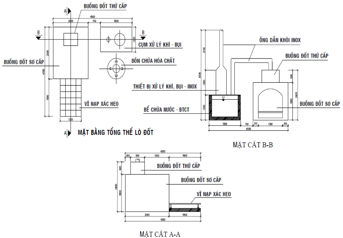
Hình 3.6.Cấu trúc lò đốt xác heo
