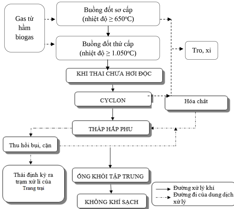
Hình 3.7. Quy trình vận hành lò đốt và xử lý khí thải trước khi thải ra môi trường
