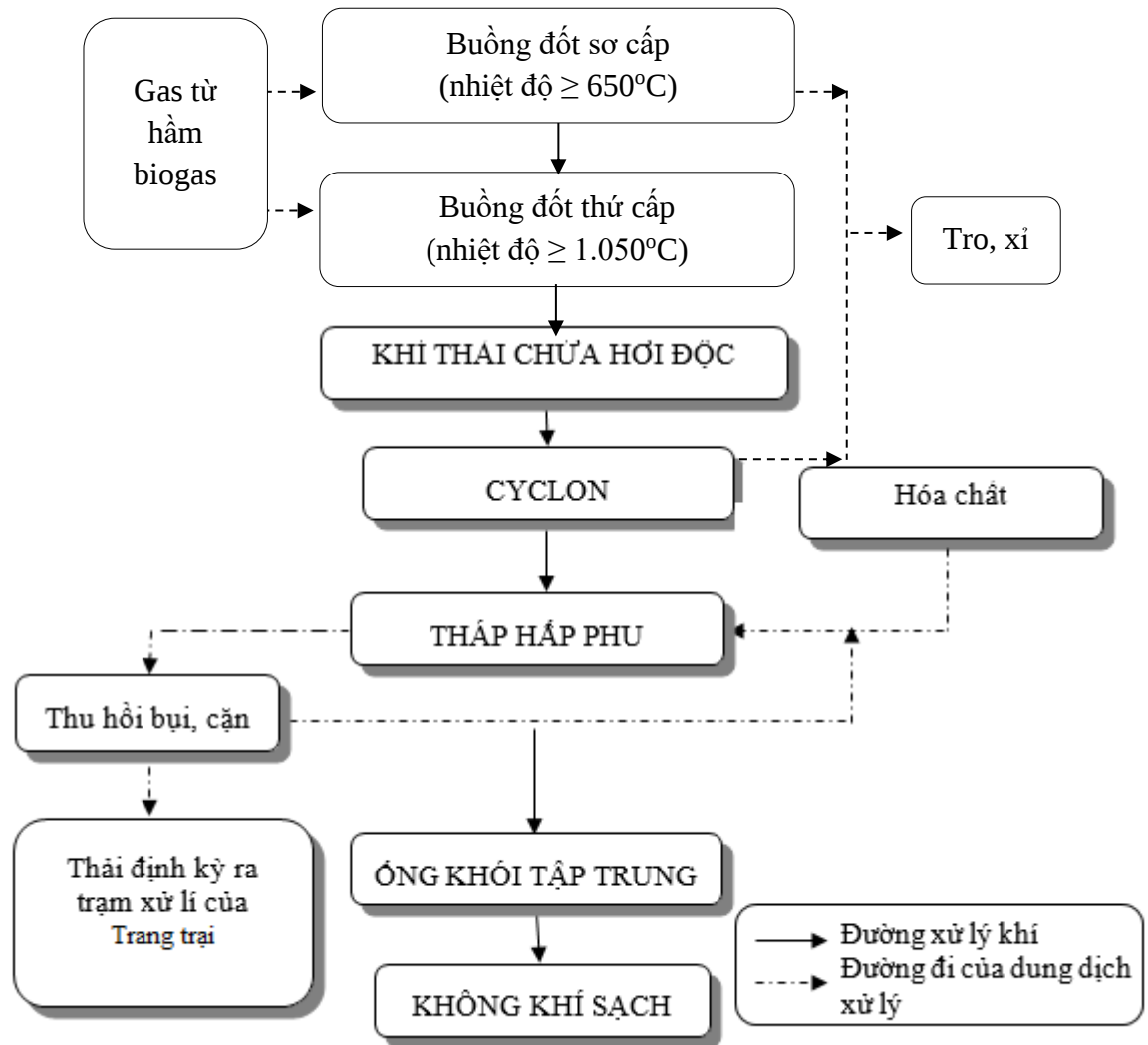
Hình 3.5. Quy trình lò đốt xác heo
