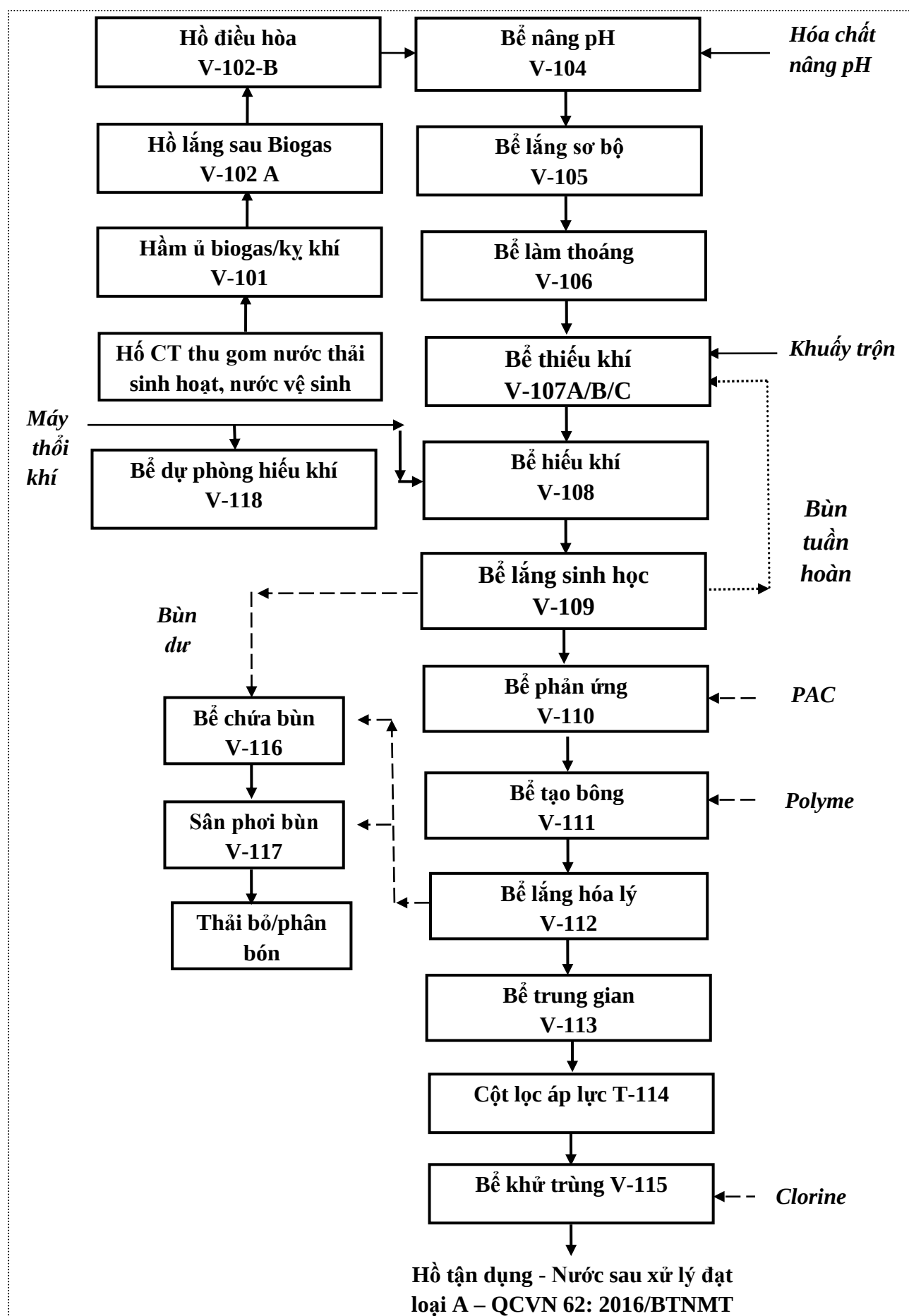
Hình 3.2. Quy trình công nghệ xử lý nước thải
