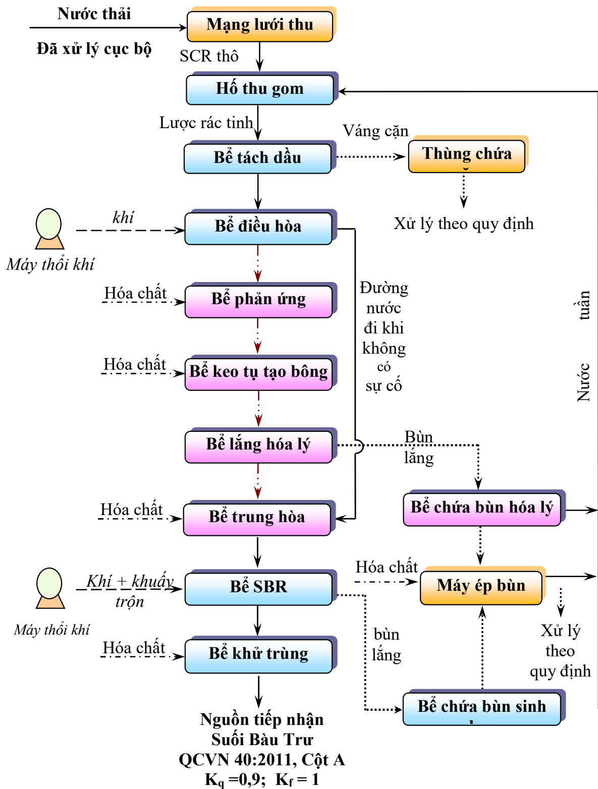
Hình 3. 2: Sơ đồ quy trình công nghệ Trạm XLNT tập trung của KCN + Hồ thu gom nước thải, tách rác
